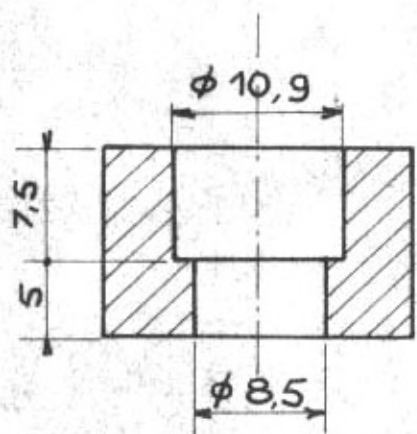
douille d'appui commune éch: 2
